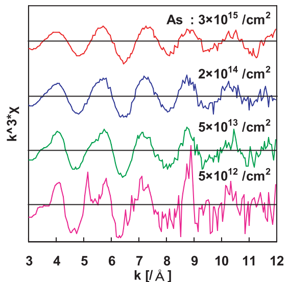
図5 抽出されたAs-K吸収端EXAFS関数
