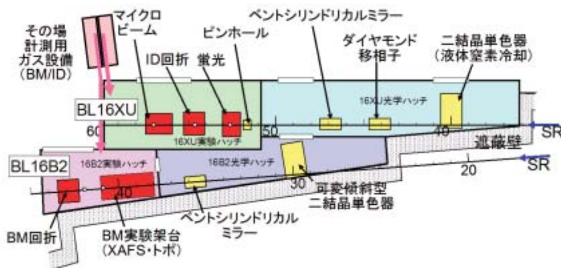
図1 BL16B2 / BL16XU全体構成図
