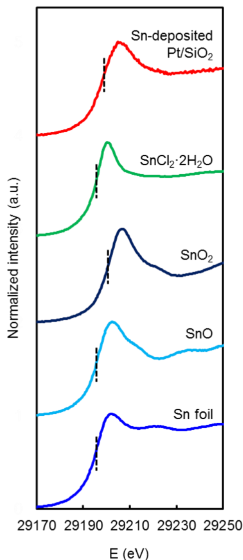
図 1. Sn foil、SnO、SnO 2 、SnCl 2 ·2H 2 O および Sn-deposited Pt/SiO 2 における Sn-K 吸収端の XANES スペクトル
