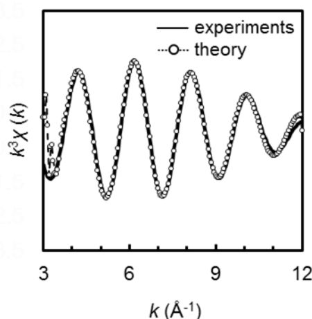
図 3. Sn-deposited Pt/SiO 2 における Sn K-edge k^3 -weighted EXAFS のカーブフィッティング (R = 1.7 Å のピークを、SnO 2 の Sn-O により解析)
