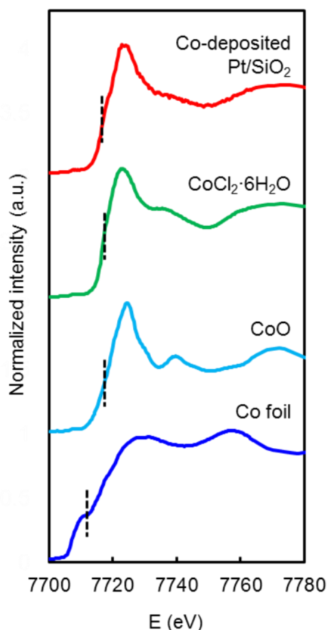
図 4. Co foil、CoO、CoCl 2 ·6H 2 O および Co-deposited Pt/SiO 2 における Co-K 吸収端の XANES スペクトル
