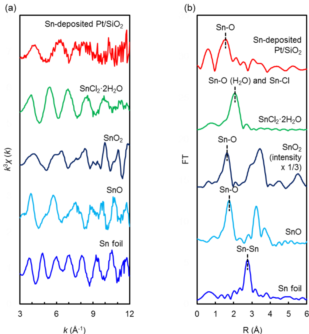
図2. Sn-K 吸収端に関する(a) EXAFS 干渉関数および(b)動径構造関数 (フーリエ変換範囲： k=3-12 \text{\AA}^{-1} )
