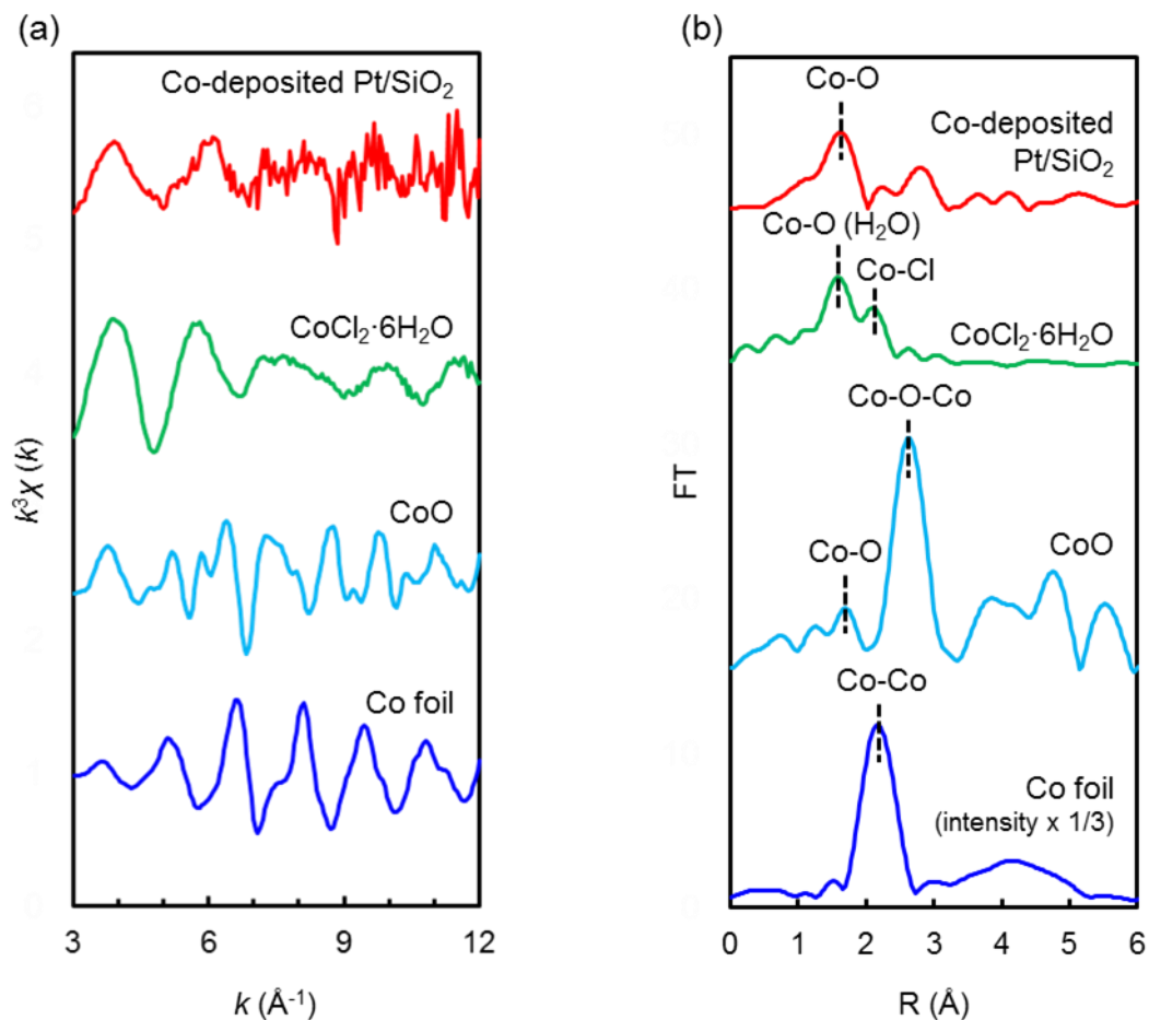
図5. Co-K 吸収端に関する(a) EXAFS 干渉関数および(b)動径構造関数（フーリエ変換範囲： k = 3 - 12 \text{ \AA}^{-1} ）
