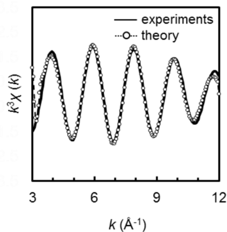
図 6. Co-deposited Pt/SiO 2 における Co K-edge k^3 -weighted EXAFS のカーブフィッティング ( R = 1.6 \text{ \AA} のピークを、CoO の Co-O により解析)
