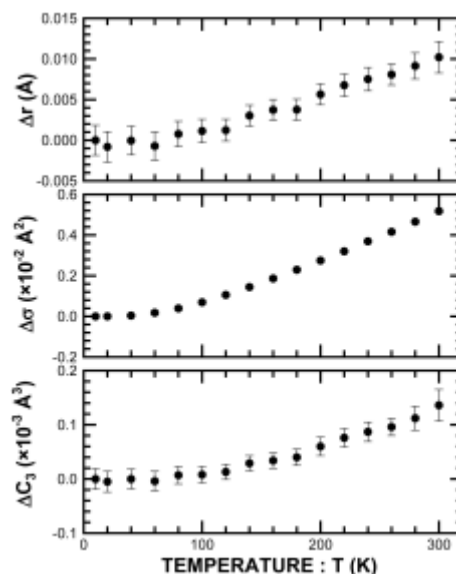
図 6. Cu 箔の最近接原子 Cu の原子間距離 r 、Debye-Waller 因子 \sigma 、C3 の温度変化 (カーブフィッティング範囲 : 1.4 \sim 2.8 \text{ \AA} 、10 K で測定したデータを基準とする)
