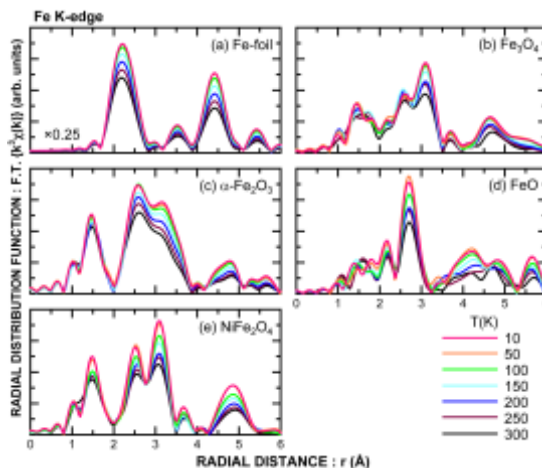
図 7. 10 K から 300 K まで変化させて測定した(a)Fe 箔、(b)Fe 3 O 4 、(c) \alpha -Fe 2 O 3 、(d)FeO、(e)NiFe 2 O 4 の動径構造関数(Fe K 端にて測定、フーリエ変換範囲：2.0～12.0 Å -1 )
