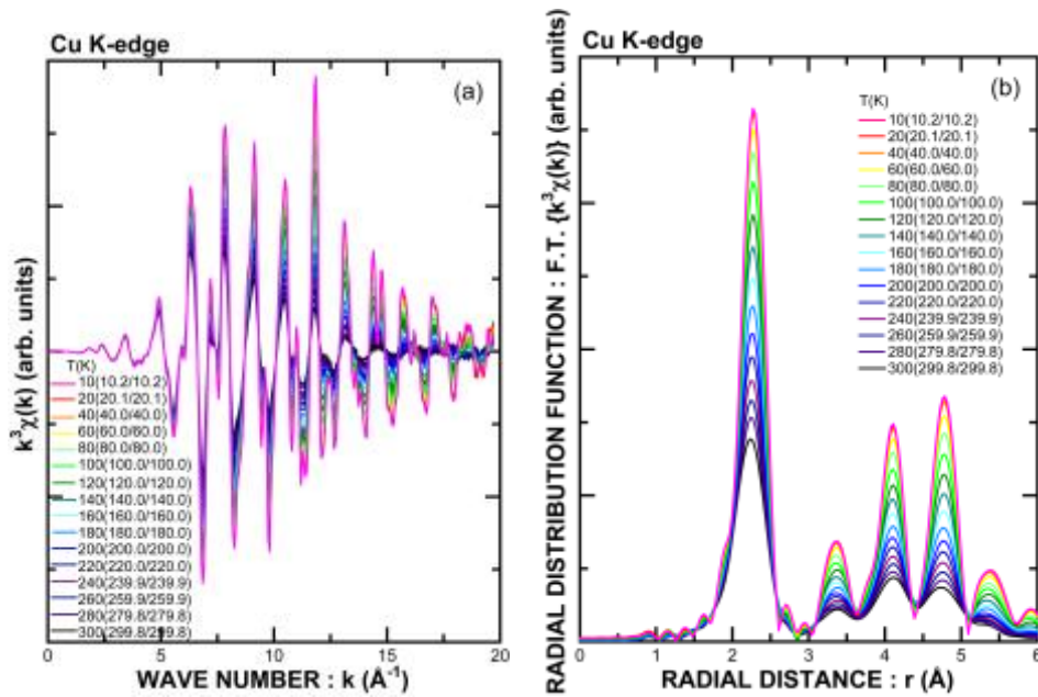
図 5. Cu 箔を 10 K から 300 K まで変化させて測定した(a)規格化 EXAFS、(b)動径構造関数 (Cu-K 端にて測定、図中の温度表記は設定値(測定開始時/終了時)を示す。フーリエ変換範囲 : 2.0 \sim 17.0 \text{ \AA}^{-1} )
