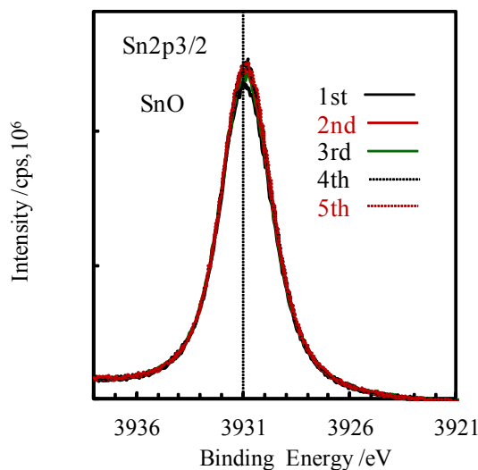
図3 SnO の光電子スペクトル経時変化
