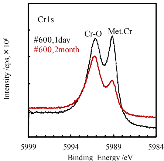
図5 Cr 1s の光電子スペクトル 脱出角度：80°,研磨1日：黒, 研磨2カ月：赤
