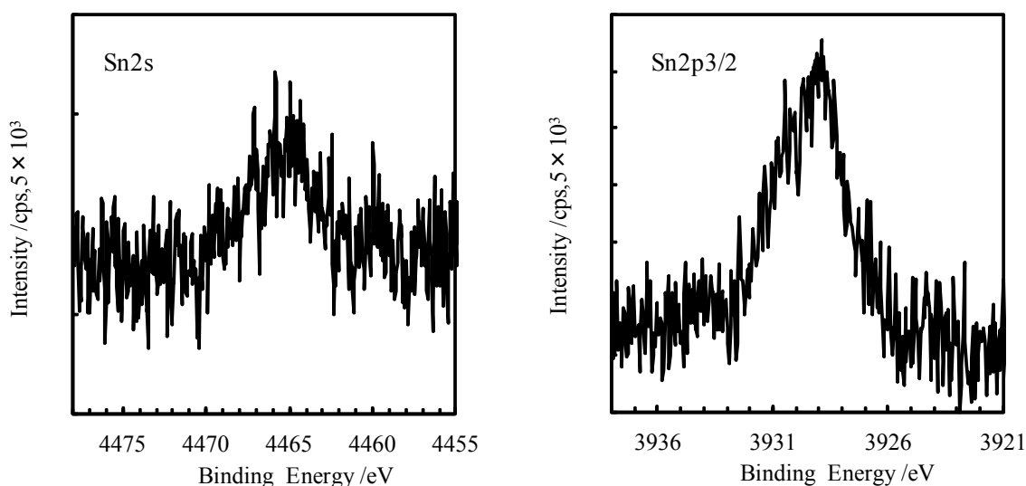
図 1 脱出角度 80°の Sn 2s と Sn 2p 3/2 の光電子スペクトル
