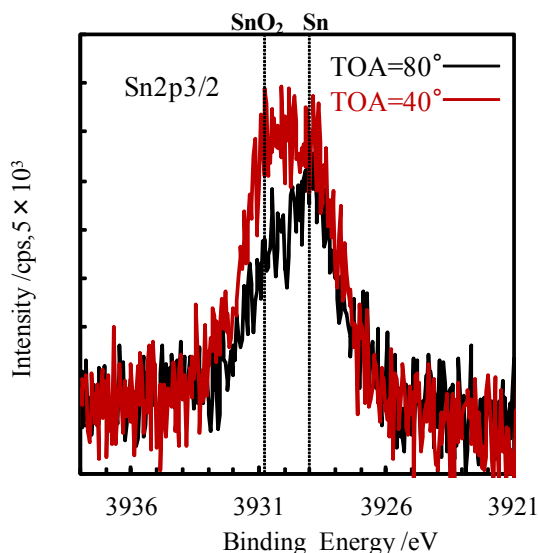
図4 Sn 2p 3/2 の角度分解スペクトル 脱出角度：80° (黒) ,40° (赤)
