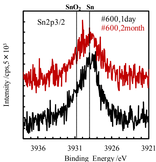
図 6 Sn 2p 3/2 の光電子スペクトル 脱出角度：40°、研磨 1 日：黒、研磨 2 カ月：赤
