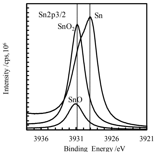
図2 標準試料の Sn 2p 3/2 光電子スペクトル
