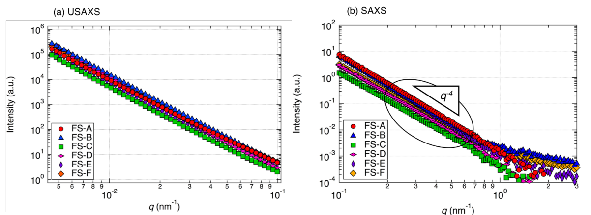
図3 (a) 放射光USAXS、(b) SAXSプロファイル
