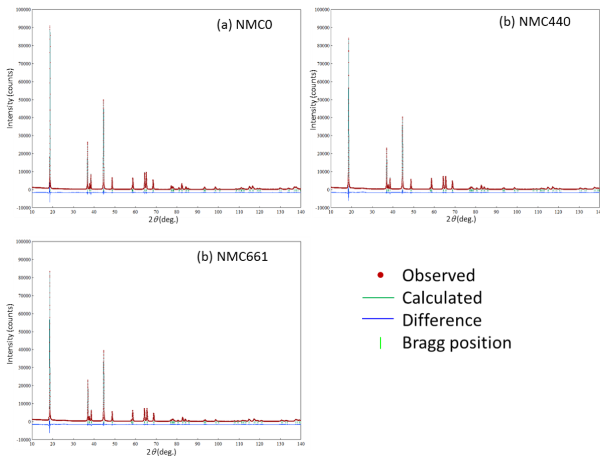
図4 実験室 X 線回折測定結果とリートベルト解析結果、(a) NMC0、(b) NMC440、(c) NMC661。
