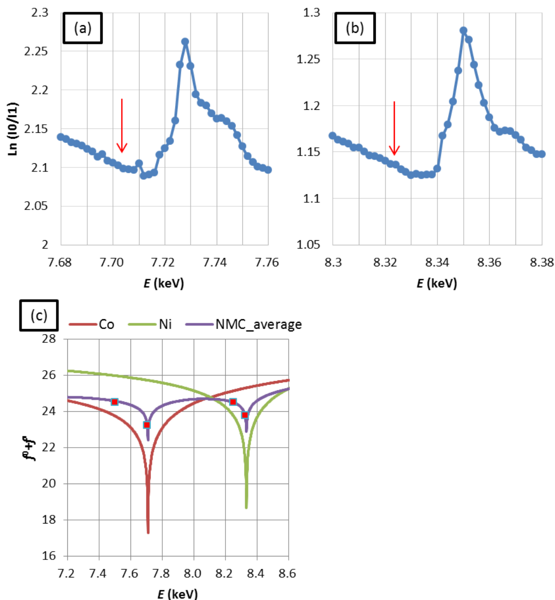
図1 (a) NMC0 の Co K 端近傍の XAFS スペクトル。試料の前のイオンチェンバーの入射強度 I_0 、透過強度 I 。 (b) NMC0 の Ni K 端近傍の XAFS スペクトル。 (a) と (b) 中の赤矢印はそれぞれ、X 線回折測定したエネルギー 7.704 keV と 8.324 keV。 (c) 孤立原子を仮定した原子散乱因子と測定エネルギーの関係。Co、Ni、および Ni-Co-Mn 3 元素(NMC)の平均値をそれぞれ実線で、実験で用いたエネルギーを NMC 3 元素の平均値上にドットで示してある。
