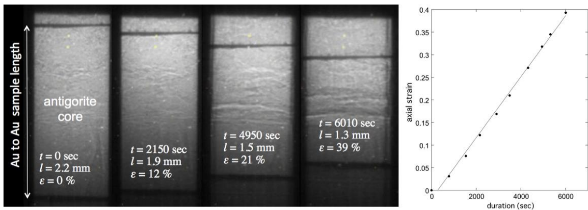
図2 一軸圧縮変形実験セルを用いたアンチゴライト円柱の変形実験 (3.1 Gpa、400°C) におけるラジオグラフィ像 (左) と軸歪みの時間変化 (右)。アンビル変位速度 300 \mu\text{m}/\text{h} 、試料の軸歪み速度 6.7 \times 10^{-5} \text{ s}^{-1} 。
